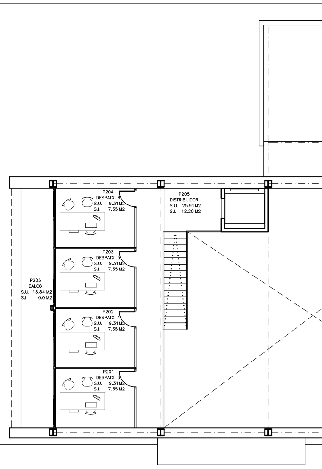
DISTRIBUCIÓ PLANTA 2
