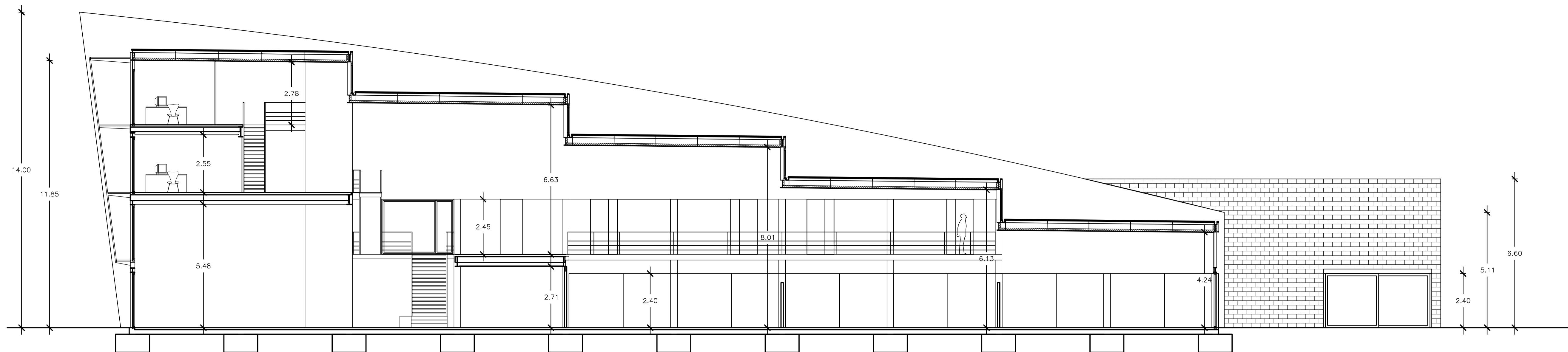
SECCIÓ SL1 (COS PRINCIPAL)
