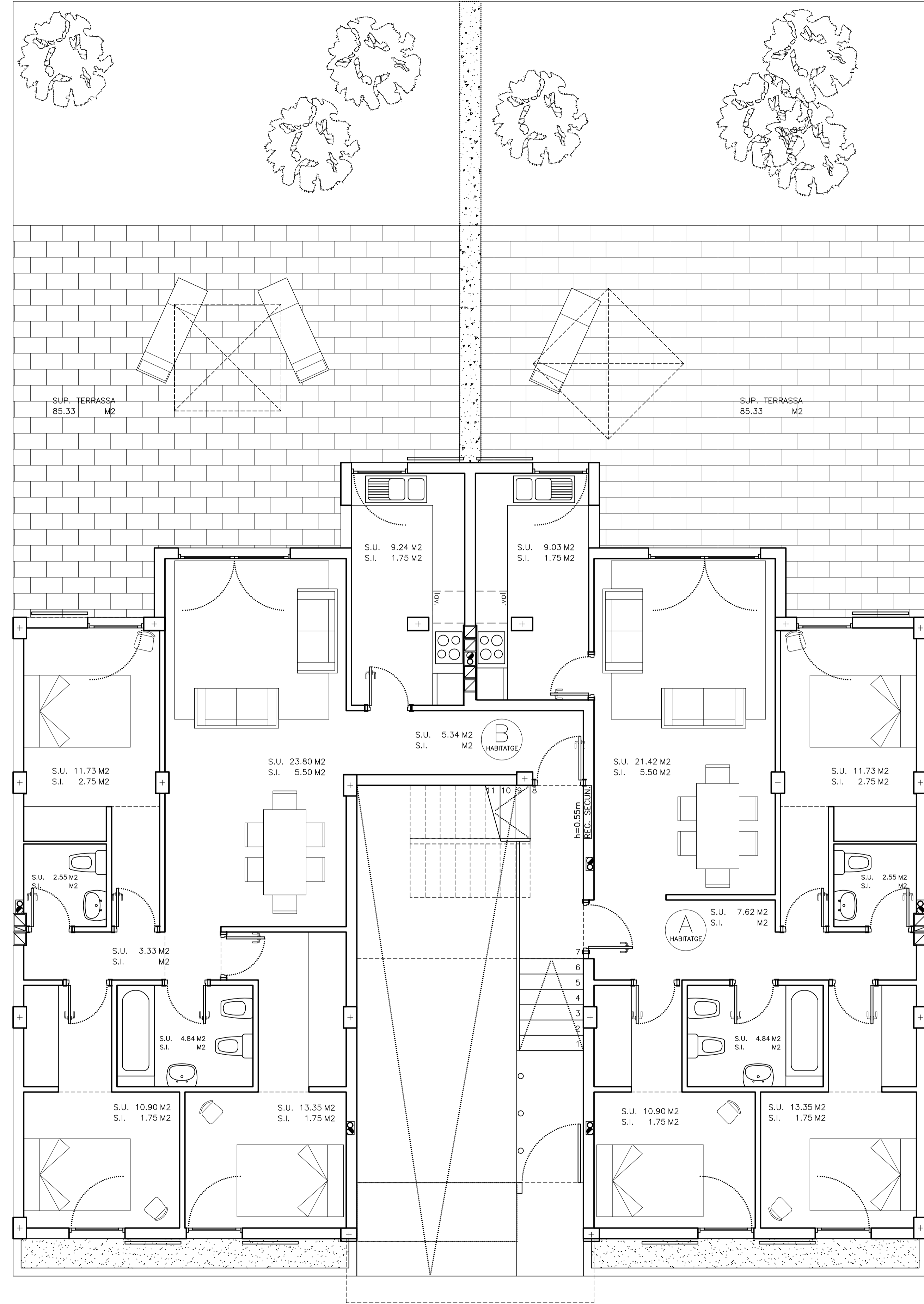
PLANTA BAIXA DISTRIBUCIÓ
