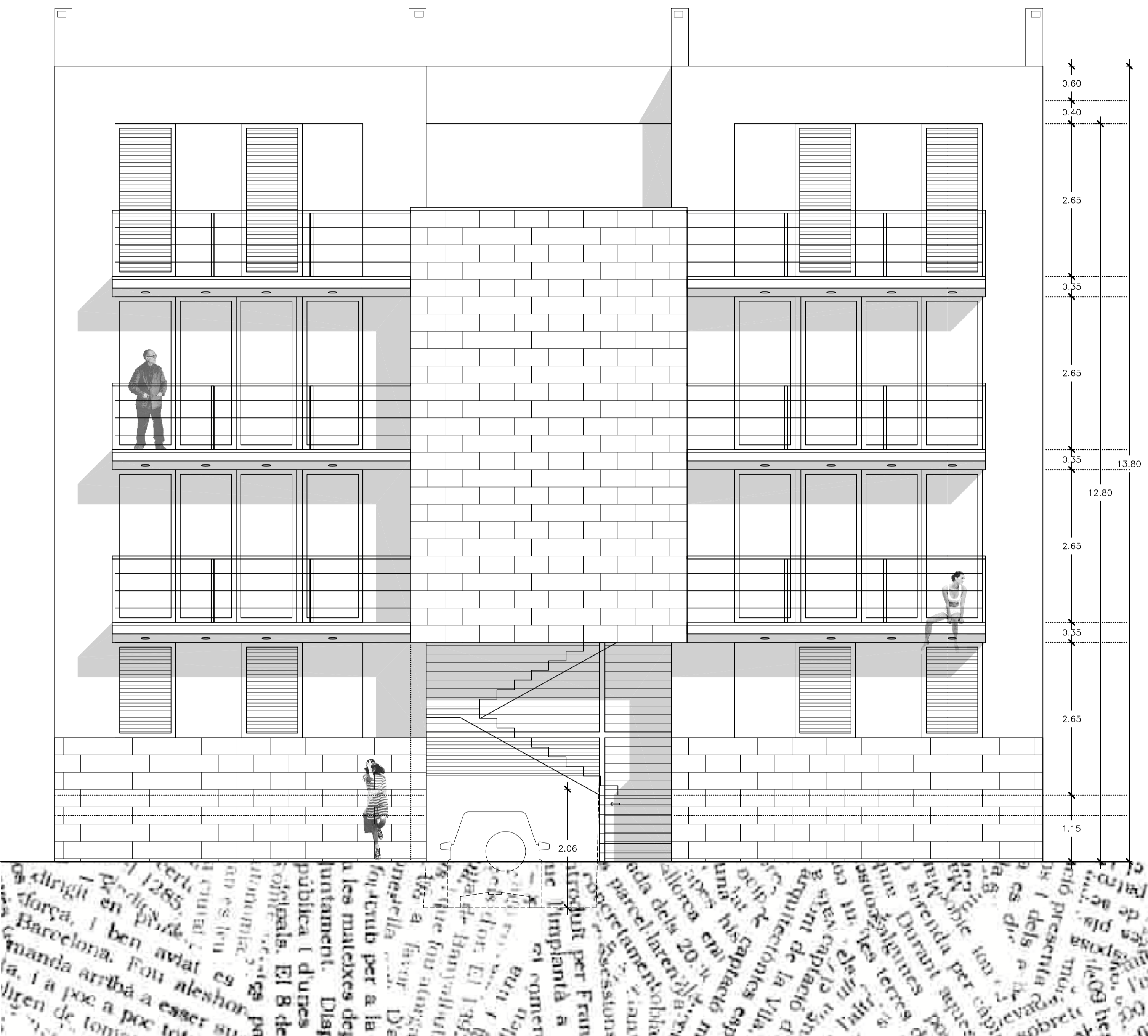
ALÇAT A (ACCÉS C/ORIENT)
